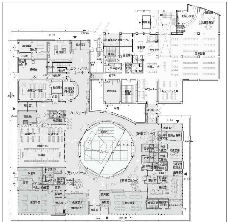
▶1階平面図
